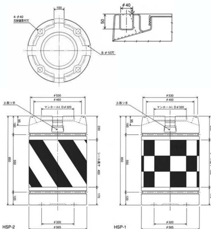
反射鏡取付穴部詳細
