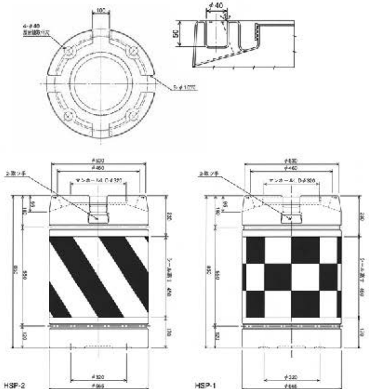
反射鏡取付穴詳細
