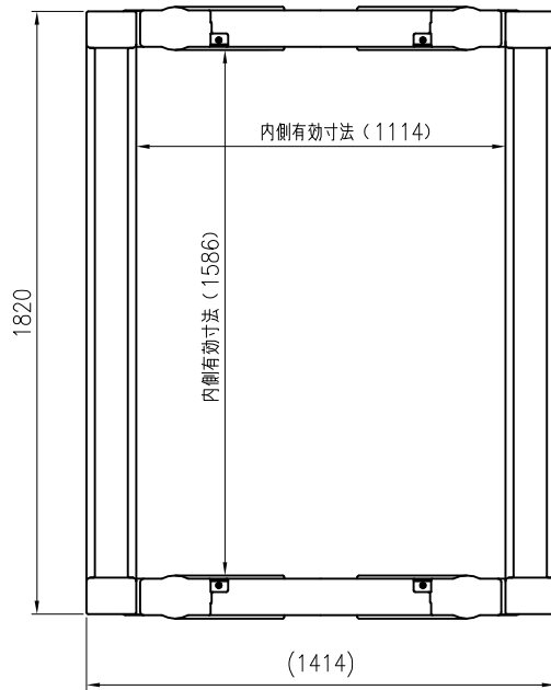
【組立平面】
