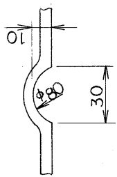
A-A断面 S=1/2
